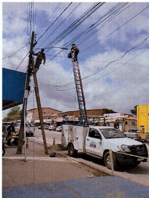
Figura 02: equipe em campo realizando substituições necessárias de Lâmpadas, cabo elétrico, conector, reator, arruela, braços com caminhonete adaptada.
