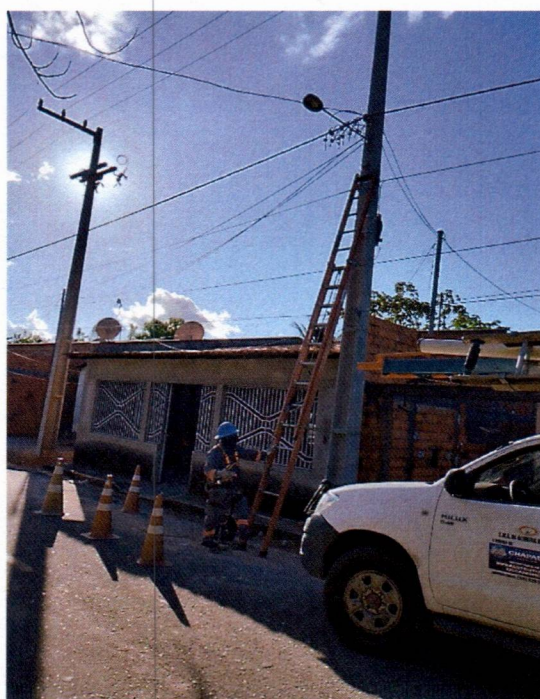
Figura 10: equipe em campo realizando substituições necessárias de Lâmpadas, cabo elétrico, conector, reator, arruela, braços com caminhonete adaptada.
