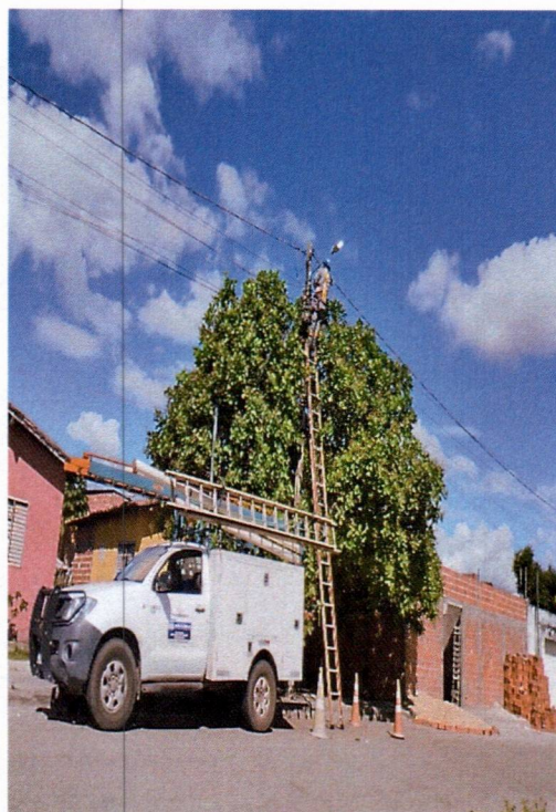
Figura 11: equipe em campo realizando substituições necessárias de Lâmpadas, cabo elétrico, conector, reator, arruela, braços com caminhonete adaptada.
