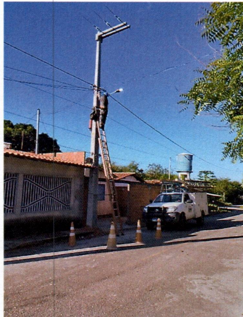
Figura 01: equipe em campo realizando substituições necessárias de Lâmpadas, cabo elétrico, conector, reator, arruela, braços com caminhonete adaptada.
