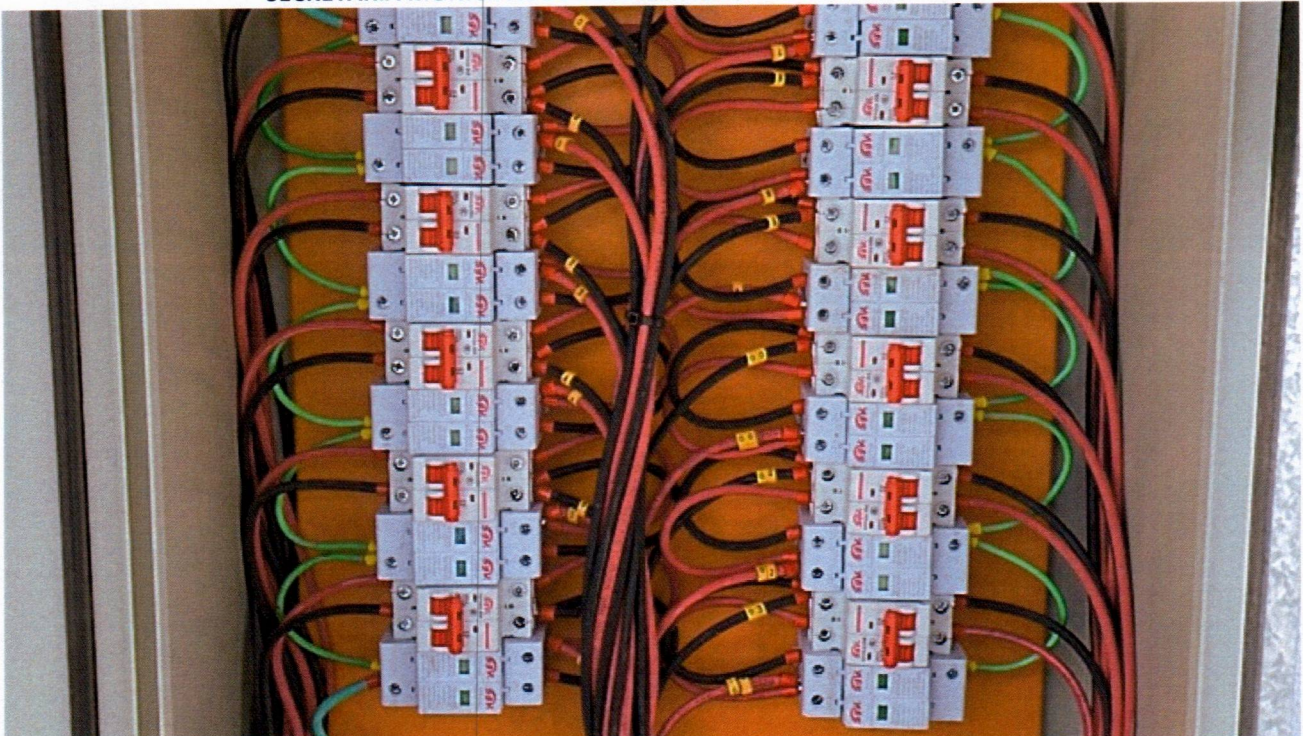
Imagem 14 – Instalações de elétricas na quadra coberta da escola UI Professor Oliveira Roma no bairro Corrente
