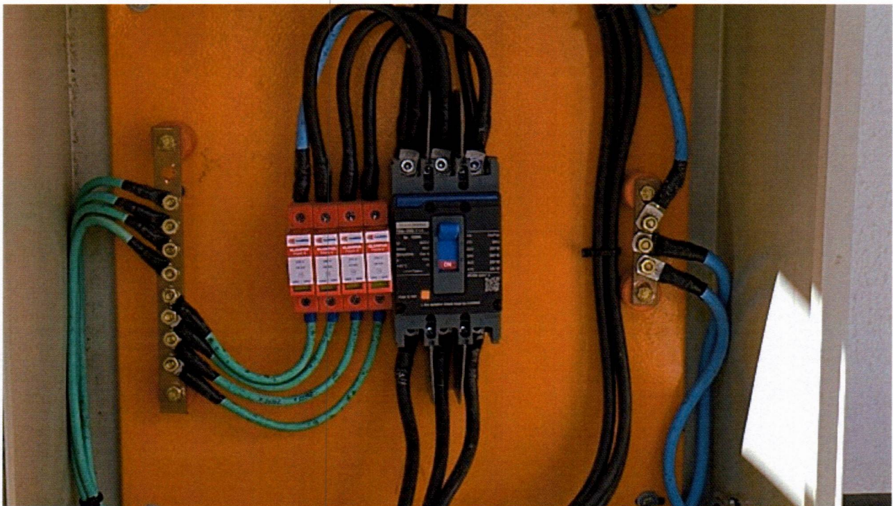
Imagem 15 – Instalações de elétricas na quadra coberta da escola UI Professor Oliveira Roma no bairro Corrente
