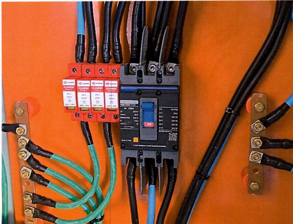
Imagem 08 – Instalações de painéis na escola U. E ANA FORTES DE MENESES
