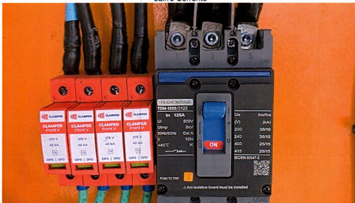
Imagem 17 – Instalações de elétricas na quadra coberta da escola UI Professor Oliveira Roma no bairro Corrente
