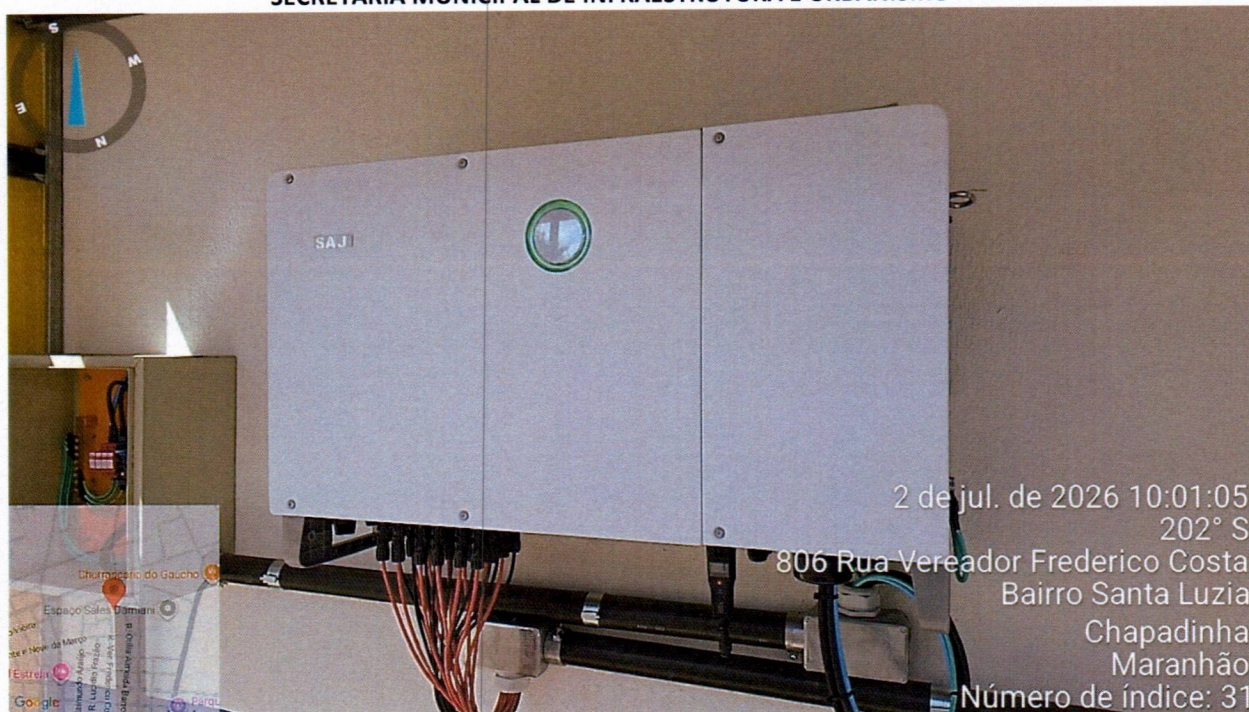
Imagem 16 – Instalações de elétricas na quadra coberta da escola UI Professor Oliveira Roma no bairro Corrente
