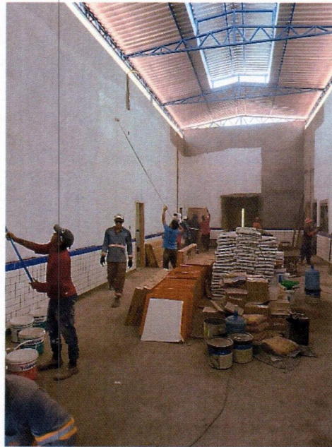
Imagem 5 – Execução da textura acrílica na parte interna do prédio.
