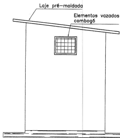
VISTA LATERAL ESCALA 1:50
