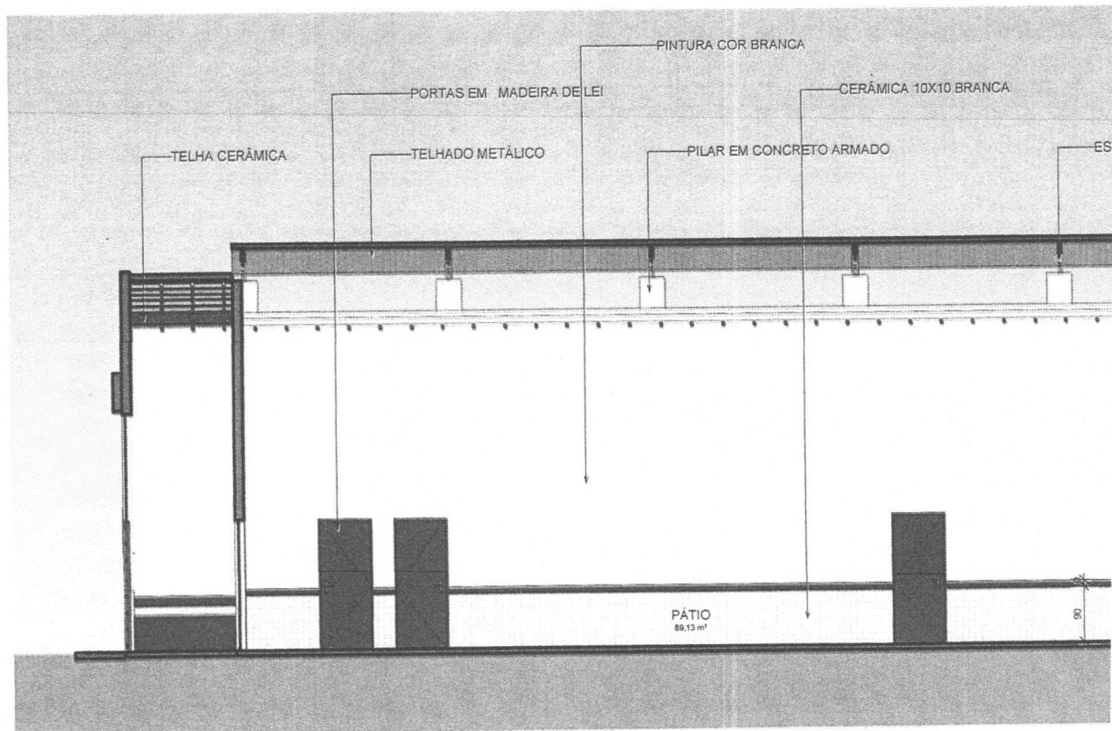
1 CORTE AA ESCALA 1:75
