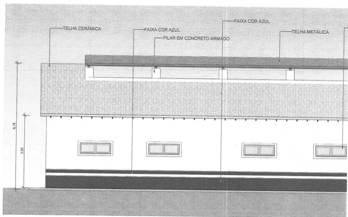
2 LATERAL ESQUERDA ESCALA 1:75
