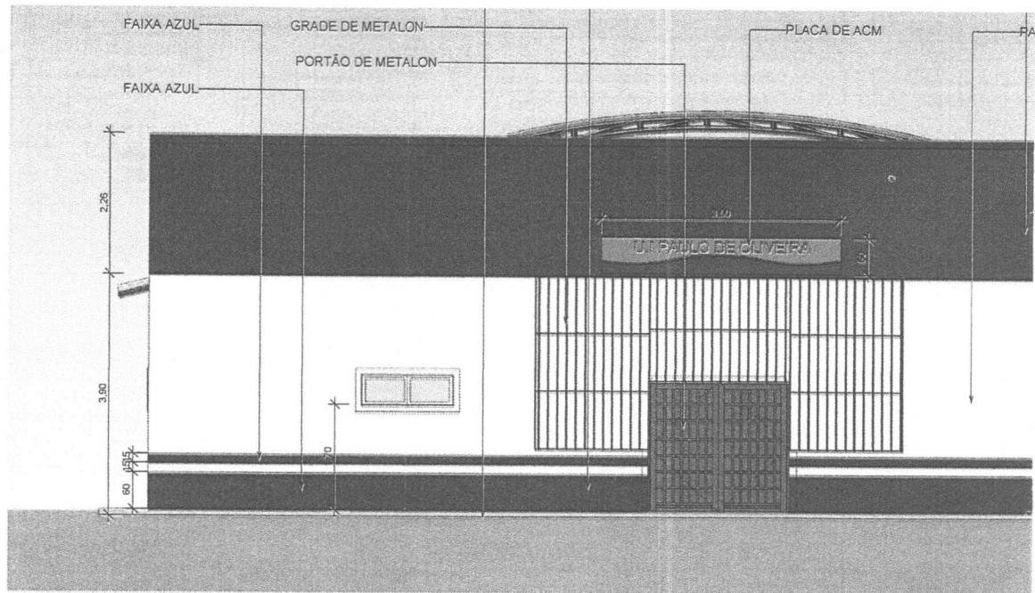
1 FRENTE ESCALA 1:75
