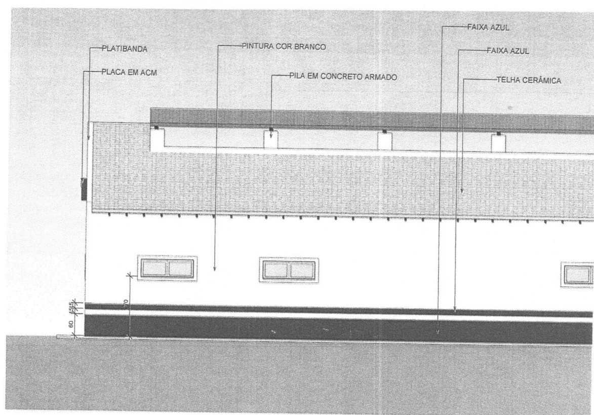
1 LATERAL DIREITA ESCALA 1:75
