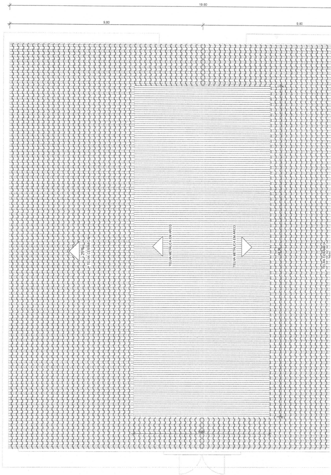
1 COBERTURA ESCALA 1:75
