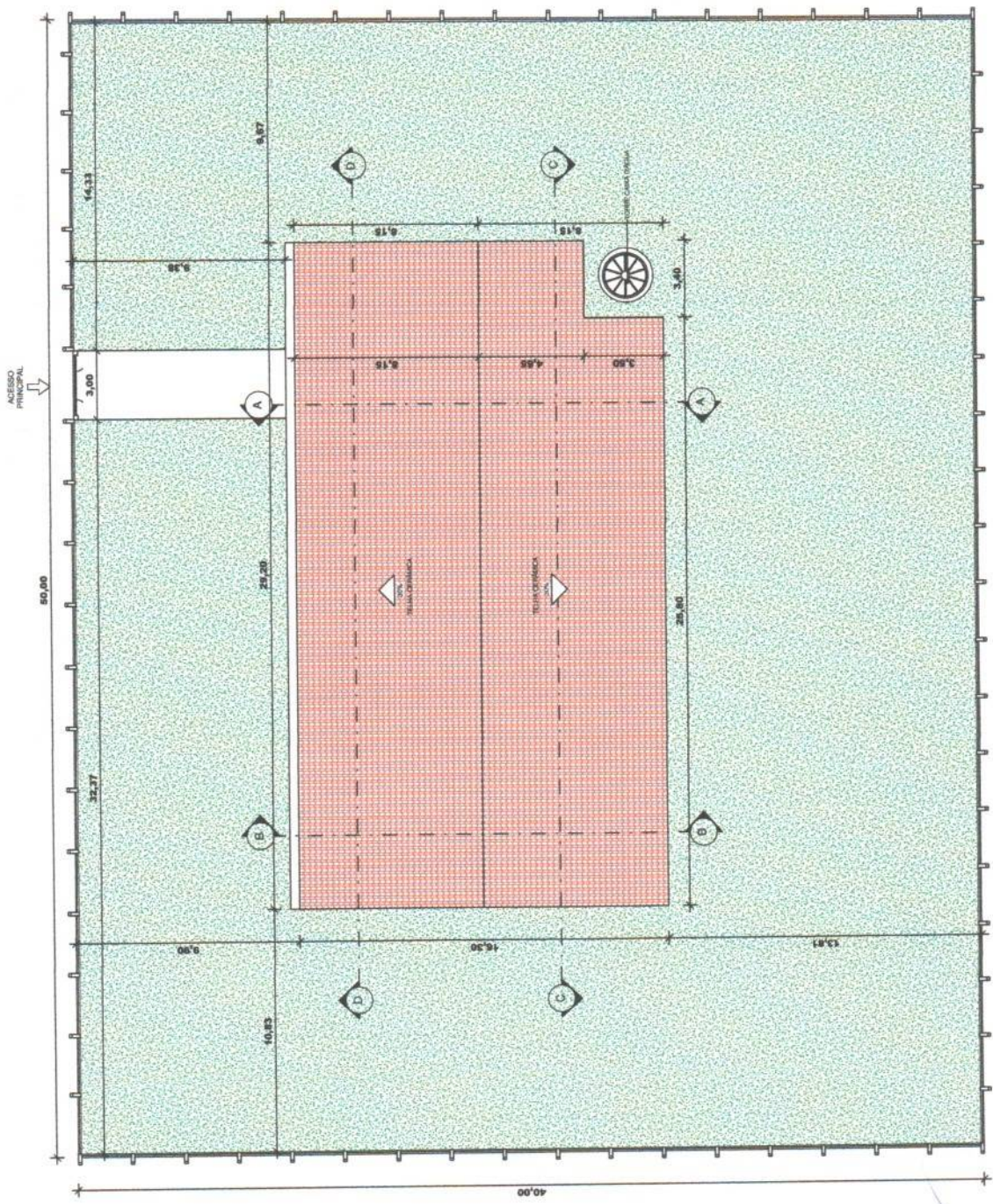
1 - IMPLANTAÇÃO COBERTURA ESCALA 1:100
