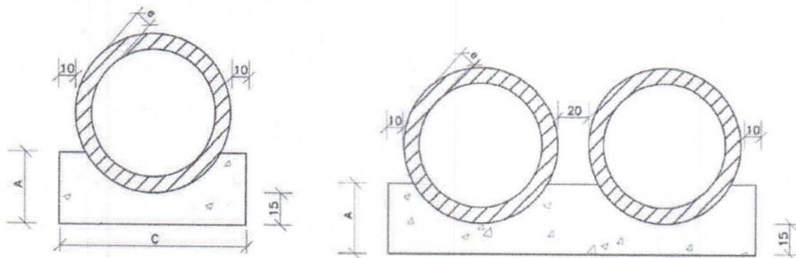
Figura 3 - Bueiro simples tubular de concreto (BSTC) e Bueiro duplo tubular de concreto (BDTC), respectivamente
