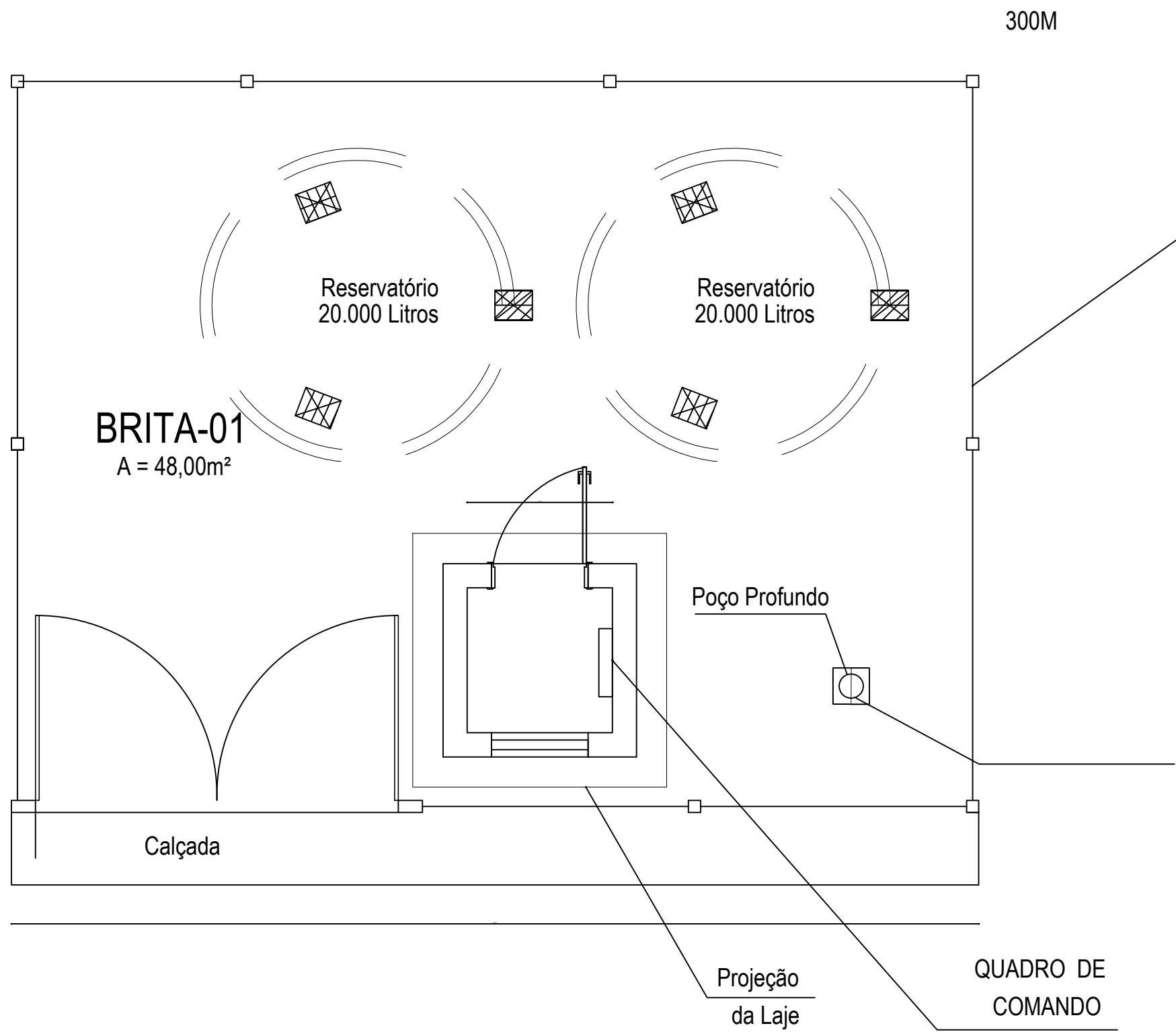
PLANTA DE DETALHES-05
