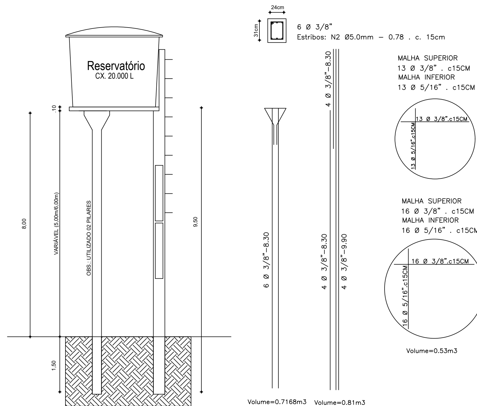
VISTA esc 1:50
