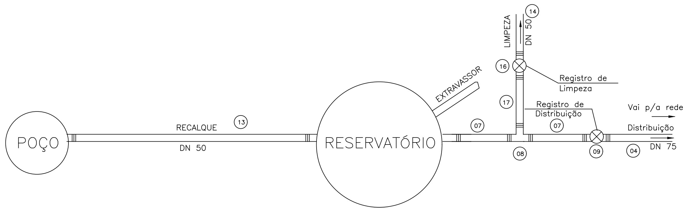
PLANTA BAIXA SEM ESCALA
