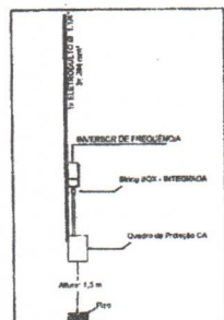
DETALHE 2 - Vista lateral do local de instalação dos Inversores
