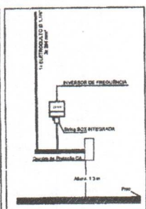
DETALHE 1 - Instalação dos Inversores
